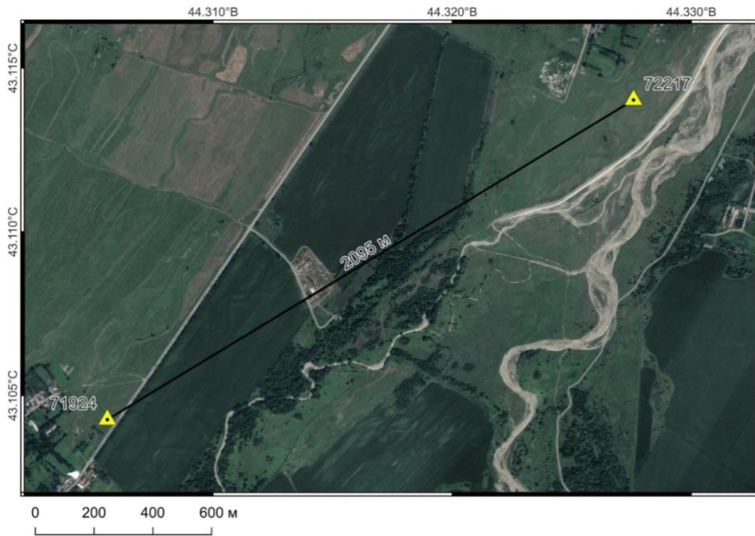
Рисунок 7.7 – Схема измерений базовой линии
