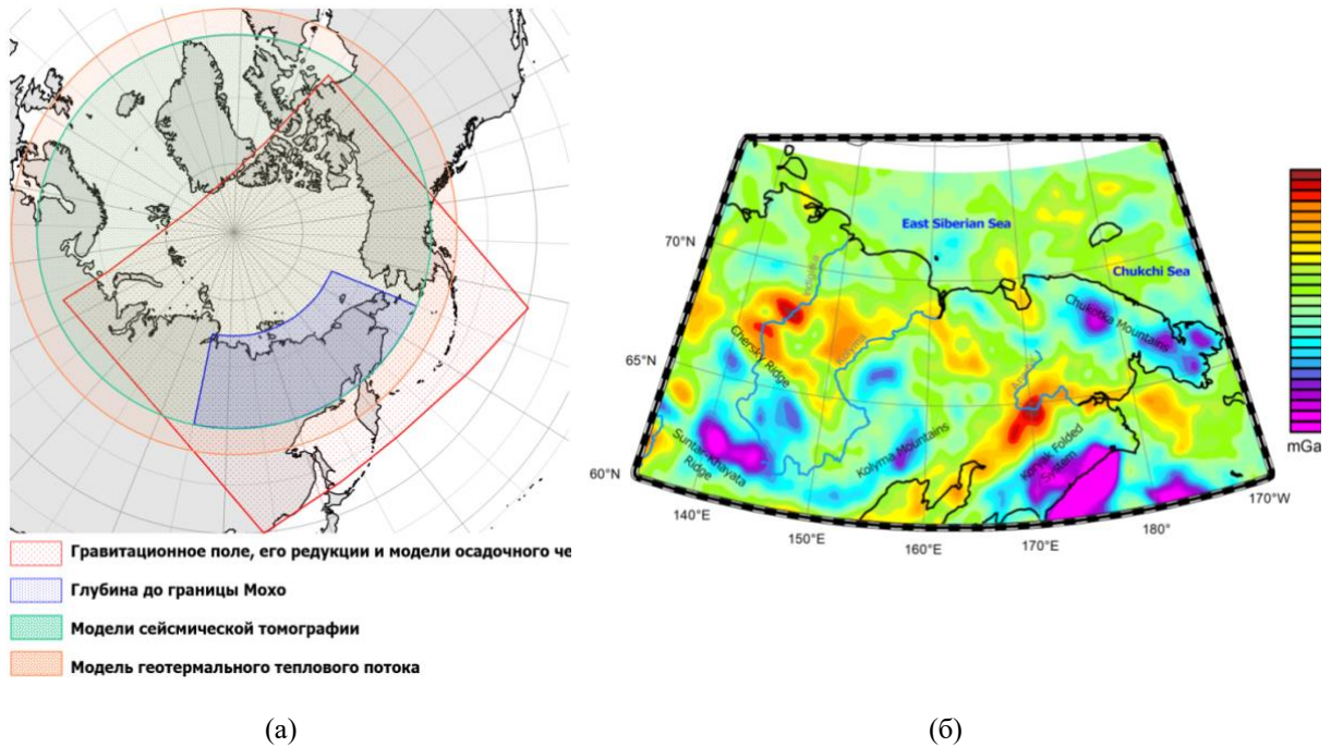
Рисунок 1.3 – Трёхмерная комплексная модель параметров литосферы и верхней мантии Арктики: а) пространственное покрытие полей; б) пример карты изостатических аномалий силы тяжести
