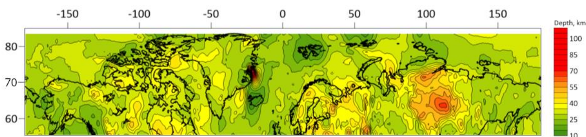
Рисунок 6.3 – Объединённая модель ГТК по данным теплового потока
