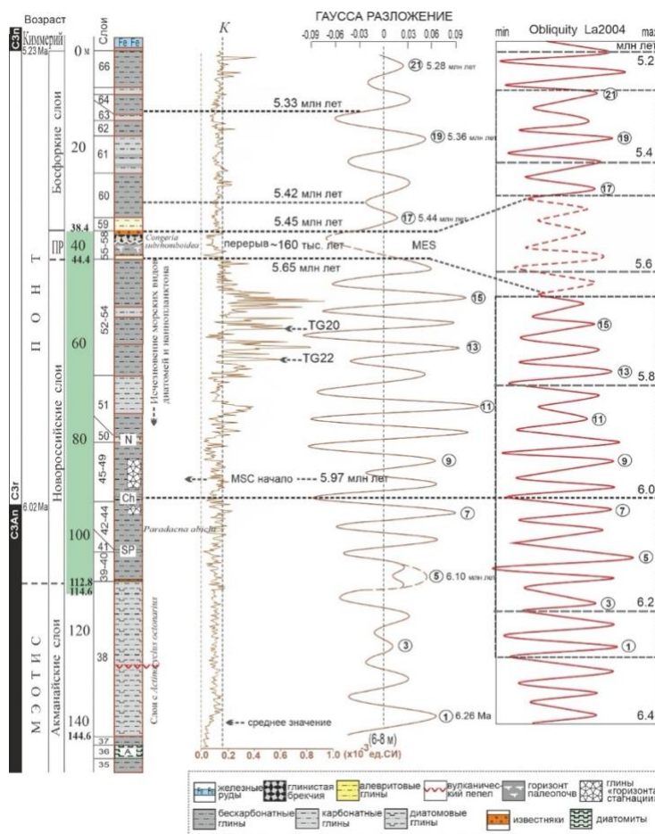
Рисунок 4.24 – AnalySeries анализ данных по магнитной восприимчивости пород понта разреза Железный Рог (Таманский полуостров). А, SP, Ch, N – прослой диатомитов (по [Radionova, Golovina, 2011]). Палеомагнитные данные по Trubikhin in [Popov et al., 1996]. Палеонтологические данные по [Popov et al., 2016]. Цифрами в кружках указаны номера циклов. ПР – портаферские слои, MSC – Мессинский кризис солёности, MES – Мессинская эрозионная поверхность, K – магнитная восприимчивость пород
