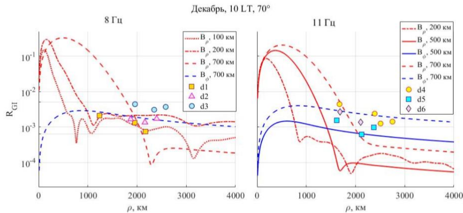
Рисунок 3.2 – Зависимость отношения амплитуды колебаний на земле к амплитуде в ионосфере от радиального расстояния: расчетные и определенные значения
