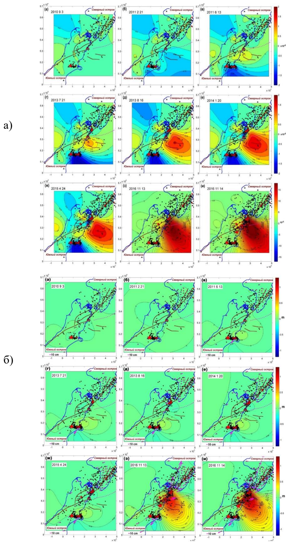
Рисунок 2.4 – Эволюция деформации дилатации (а) и горизонтальных и вертикальных движений (б) в связи в связи с землетрясениями в Новой Зеландии 2008–2021 гг.
