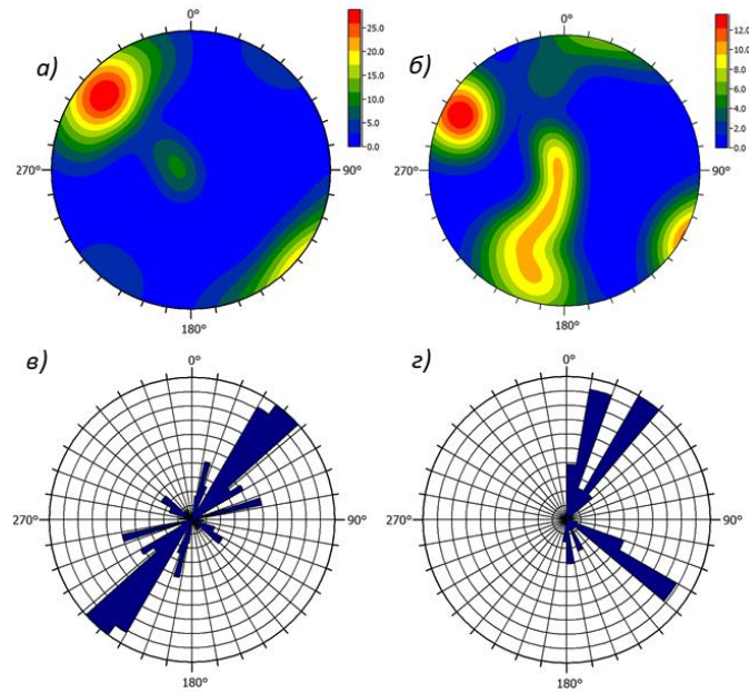
Рисунок 2.9 – Стереограммы трещиноватости пород в зоне динамического влияния Муратовского разлома (а) и в зоне динамического влияния Безымянного разлома (б), роза-диаграмма трещиноватости в зоне динамического влияния Муратовского разлома (в) и в зоне динамического влияния Безымянного разлома (з)
